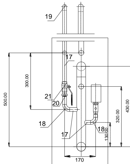
PRESEK A-A
