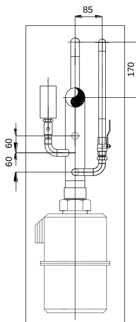
PRESEK A-A
