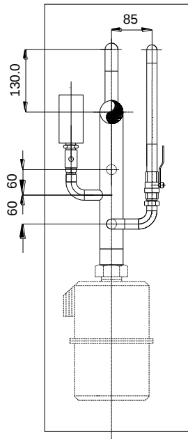
PRESEK A-A
