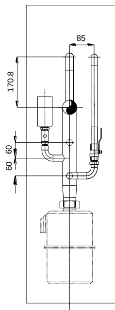
PRESEK A-A
